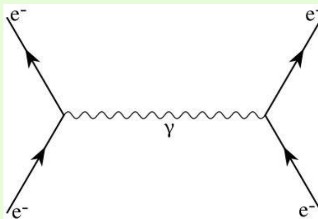
Een Feynmandiagram gebruikt in de QED: interactie tussen twee elektronen door middel van een foton
