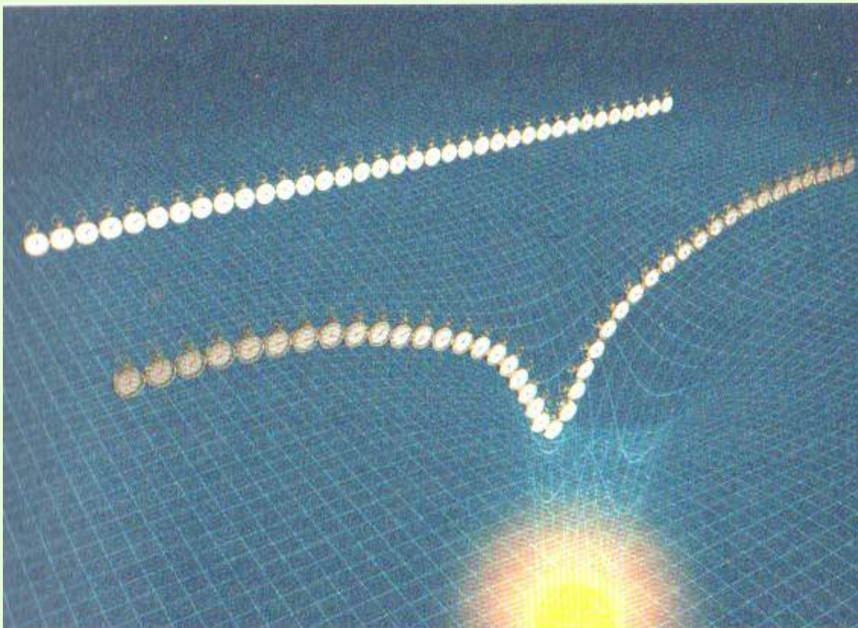
Materie en energie krommen de tijd, waardoor de tijdsdimensie zich 'vermengt' met de ruimtedimensies
